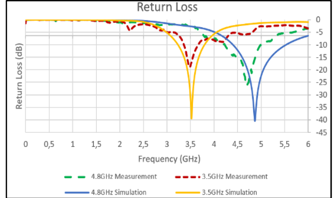
Fig. 6. Return Loss
